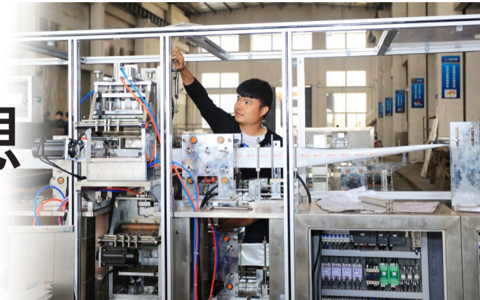
大伟机械研发的全自动面膜包装机
