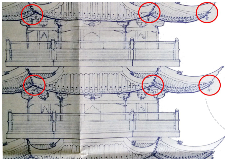
1988年工程图上的套兽所在部位
