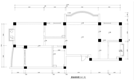
原始户型图
