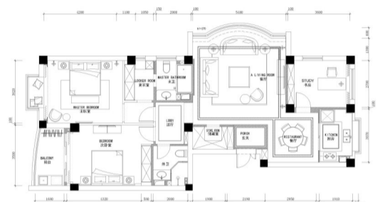
平面设计图
