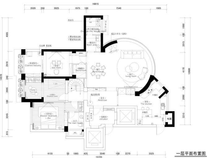
一层平面布置图
