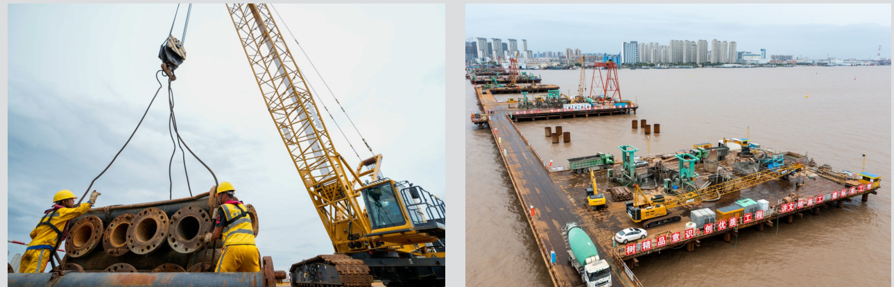
9月13日 ,省重点工程中交路建永宁大桥项目施工现场 施工人员忙着加固和转移设施设备 ,做好防御台风 梅花 工作。
